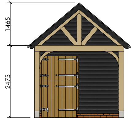
Elevation A
